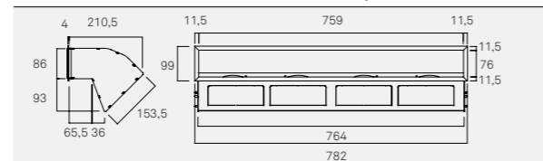
D1015 Difusor de salida de aire cuádruple
