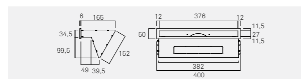
D1005 Difusor de salida de aire doble
