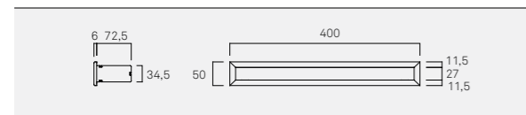
D0005 Difusor de entrada de aire doble
