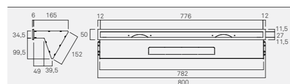
D1010 Difusor de salida de aire triple
