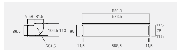
D0015 Difusor de entrada de aire cuádruple
