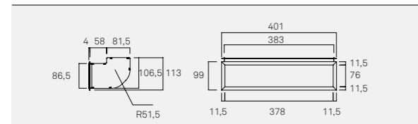
D0007 Difusor de entrada de aire doble estrecho
